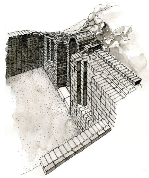
Figura 5. Dibujo de la fachada de adobe de la tumba de Djehutynefer. Dibujo realizado por Carlos Cabrera / © Proyecto Djehuty.
