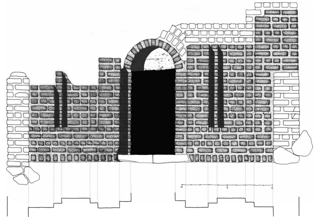
Figura 4. Dibujo de la fachada de la tumba de Djehutynefer cuya construcción imita la fachada de palacio. Dibujo realizado por Carlos Cabrera / © Proyecto Djehuty.
